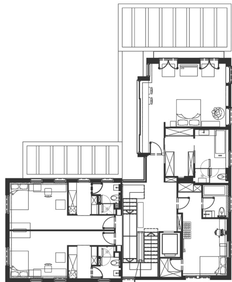
קומה ראשונה
